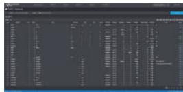
금형정보등록
