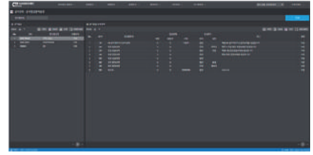
설비점검항목등록
