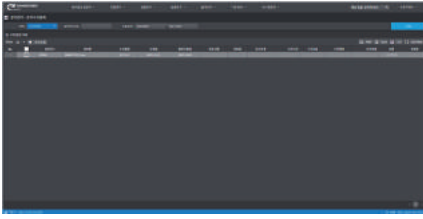
설비수리등록
