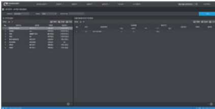
설비정기점검등록
