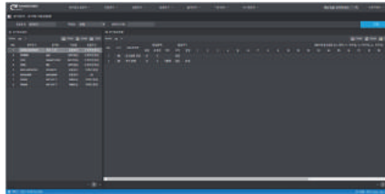
설비정기점검현황
