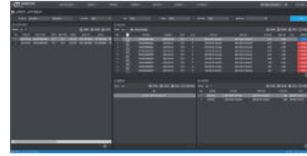
실적보정등록
