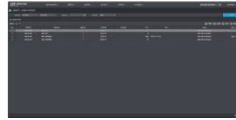
금형타수이력등록
