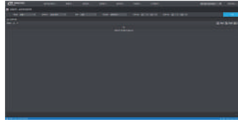
설비게더링이력
